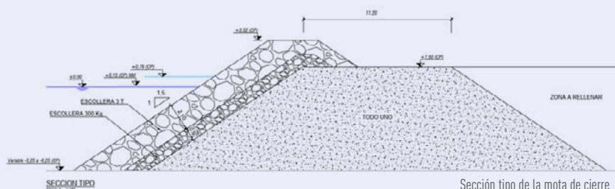
Sección tipo de la mota de cierre
