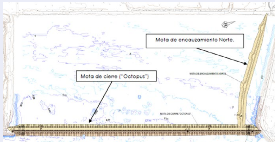
Planta general de actuaciones
