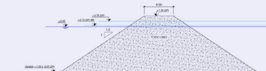
Sección tipo de la mota de encauzamiento
